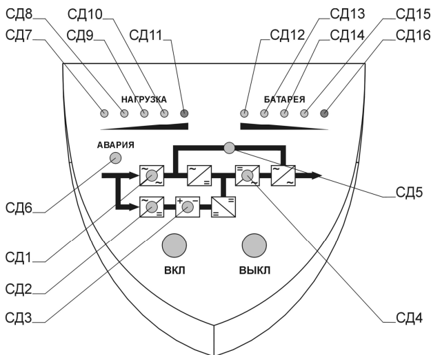
Рис. 1 Передняя панель блока ИБП
